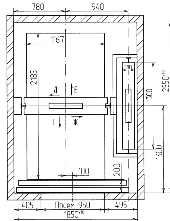
План шахты
