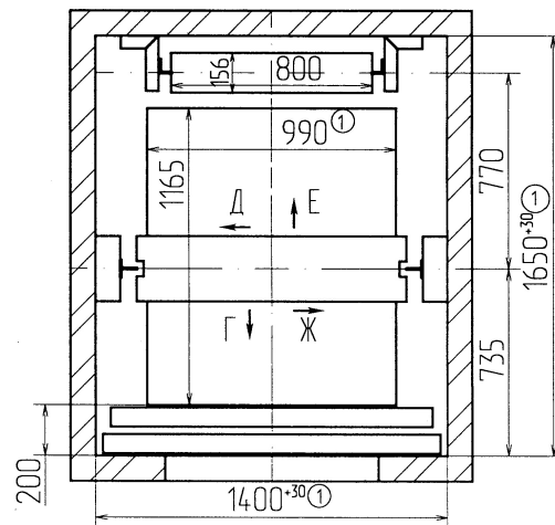
План шахты
