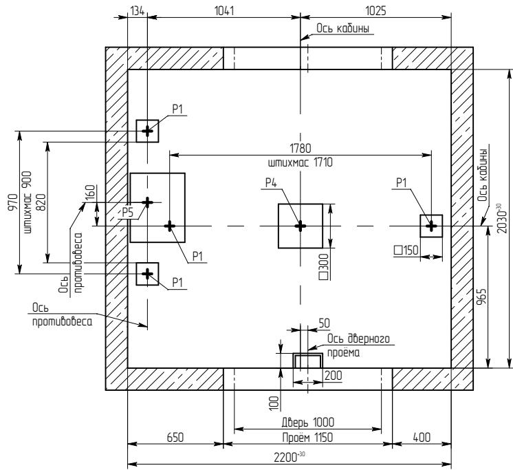
Б - Б (1:25) (1)
