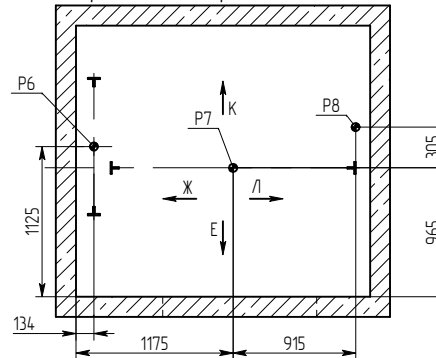
Схема расположения монтажных крюков над лифтовой шахтой
