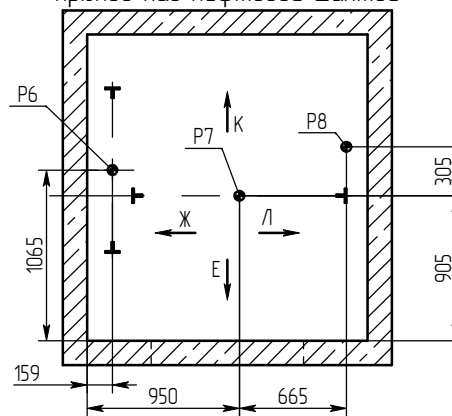
Схема расположения монтажных крюков над лифтовой шахтой
