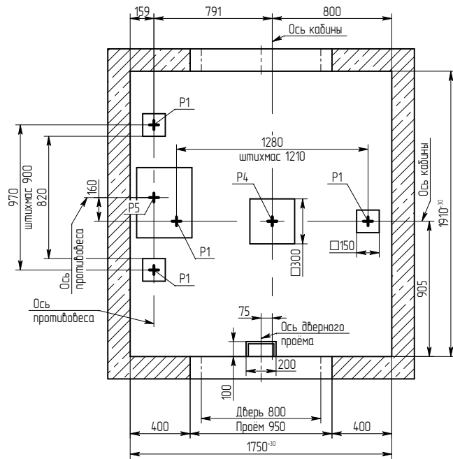
Б - Б (1:25) (1)
