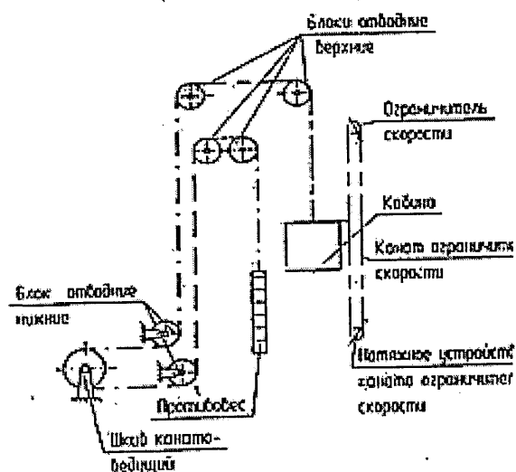
Кинематическая схема лифта (полиспастная подвеска)
