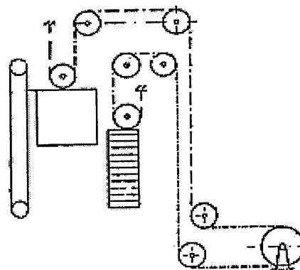
Кинематическая схема лифта (полиспастная подвеска)
