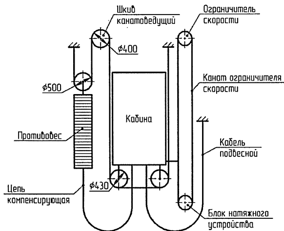
Кинематическая схема лифта
