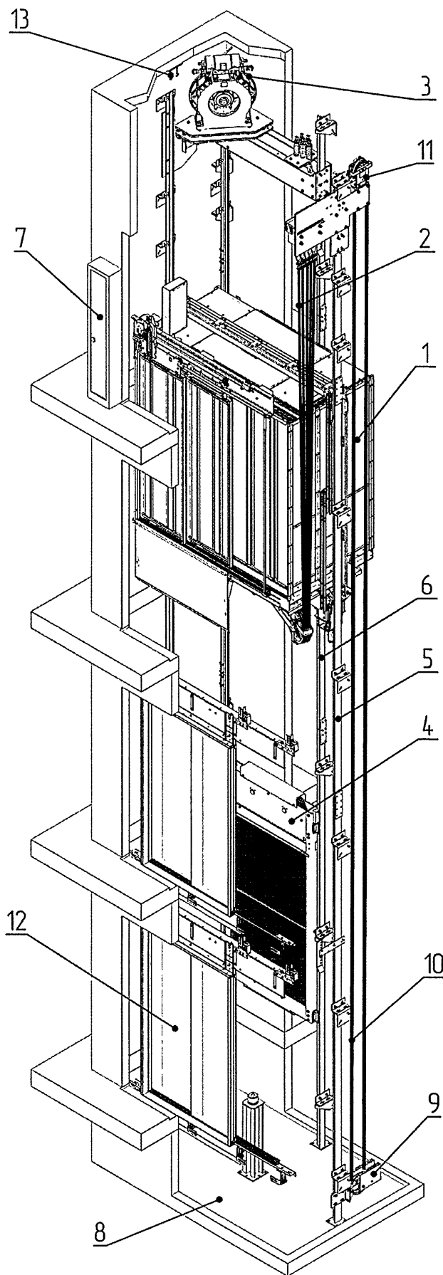
Рис. 2 Лифт пассажирский с задним противовесом
