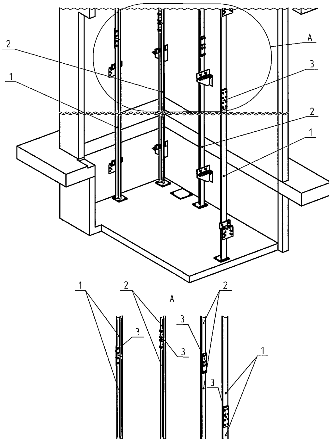
Рис 19 Установка направляющих лифта с задним противовесом
