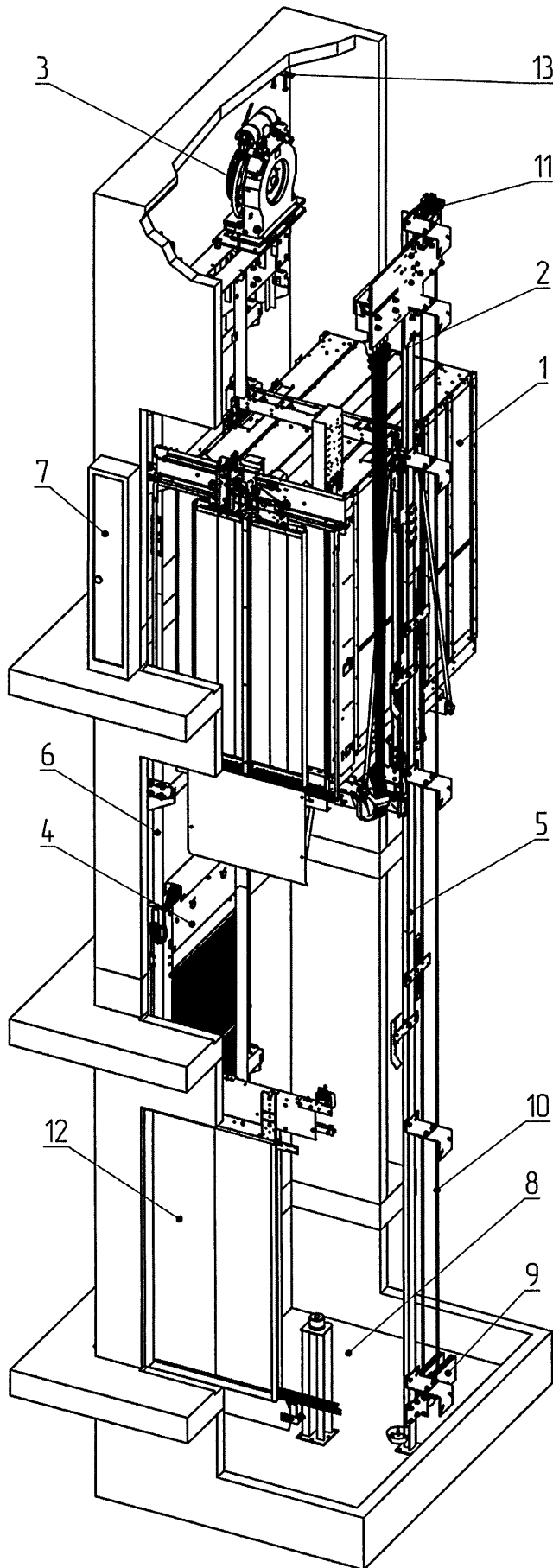
Рис. 1 Лифт пассажирский с боксовым противовесом
