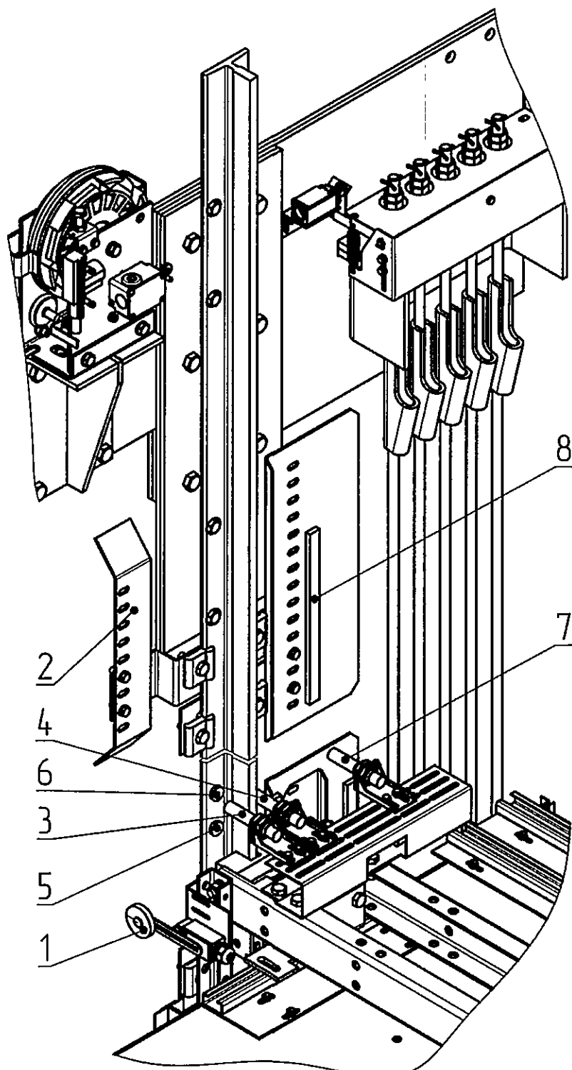
Рис. 24 Шунты, датчики, "переспуск-переподъём"
