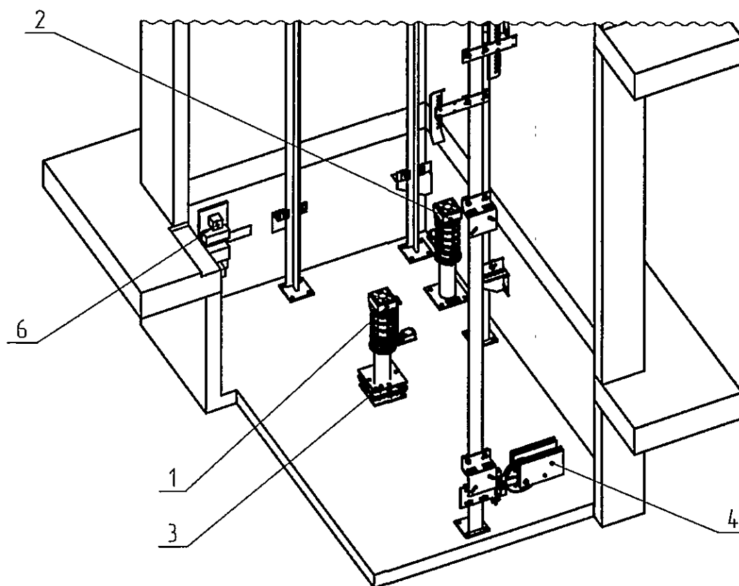
Лифт с задним противовесом
