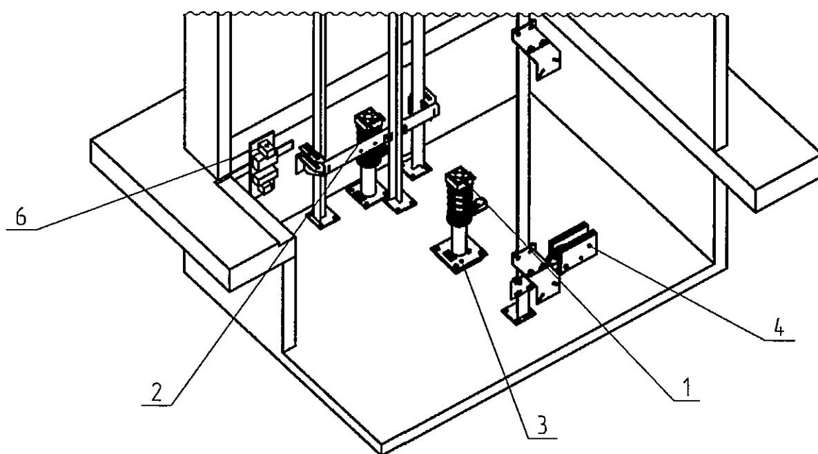
Рис 4 Оборудование прямка лифта с номинальной скоростью более 1 м/с Лифт с боковым противовесом
