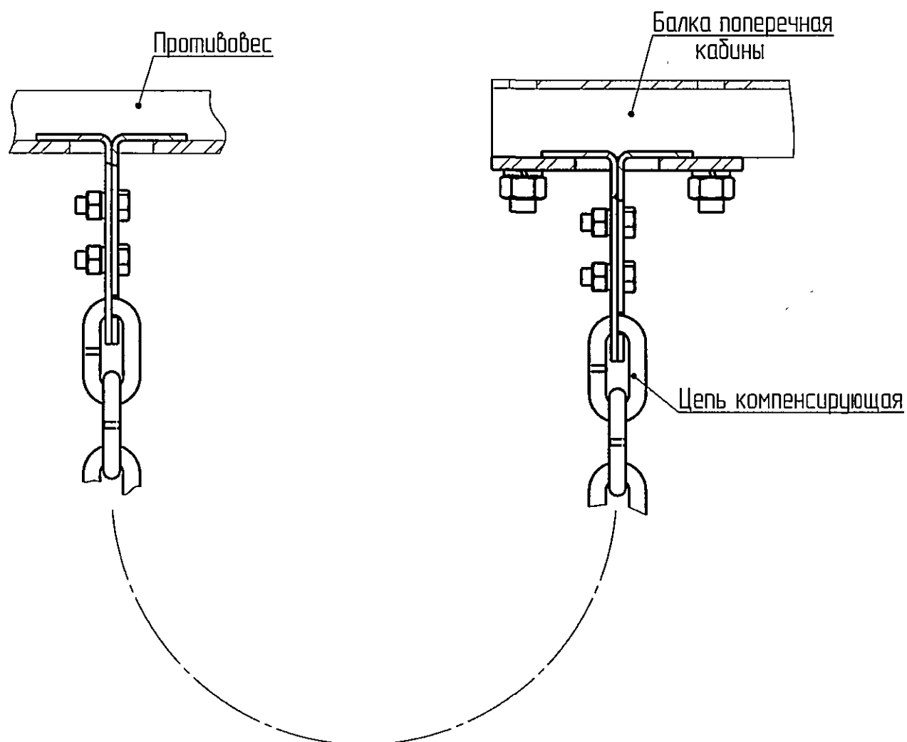
Рис. 25 Установка компенсирующей цепи
