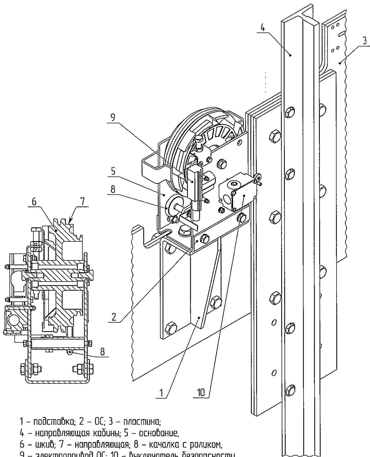
Рис 21 Установка ограничителя скорости
