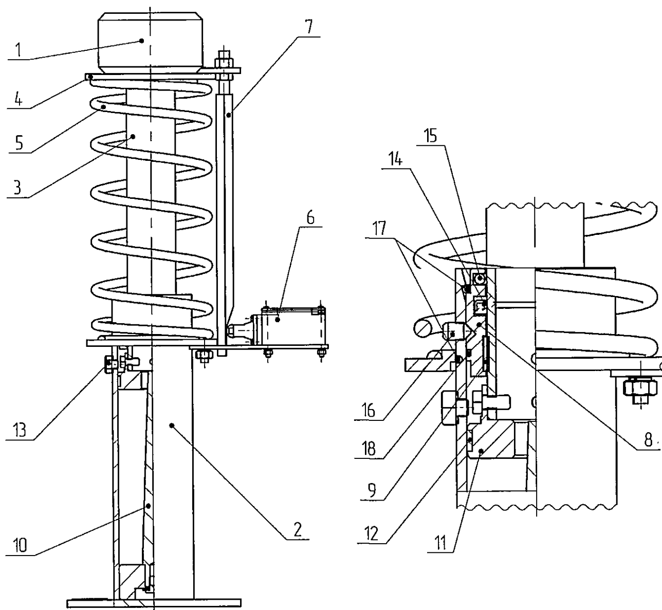
Рис 5 Буфер гидравлический
