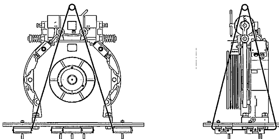
Лебёдка лифта с задним противовесом
