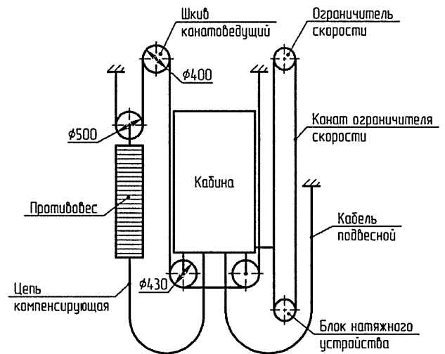
Кинематическая схема лифта
