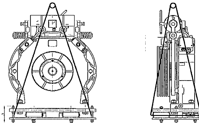
Лебёдка лифта с боковым противовесом
