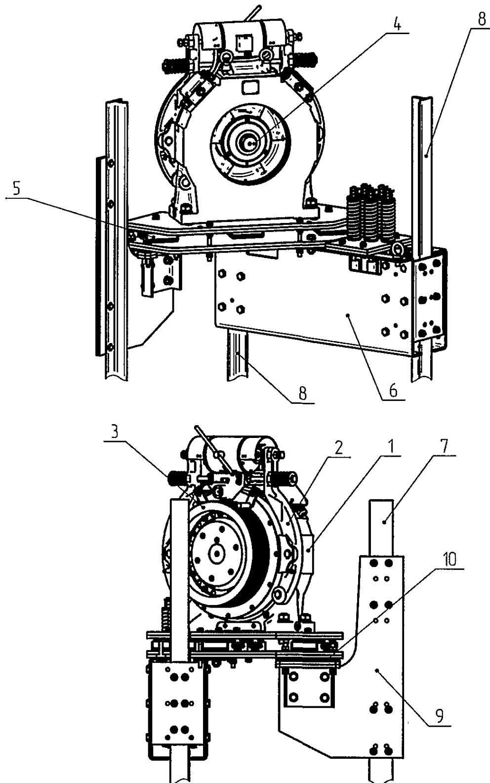
Рис. 9 Лебёдка лифта с задним противовесом
