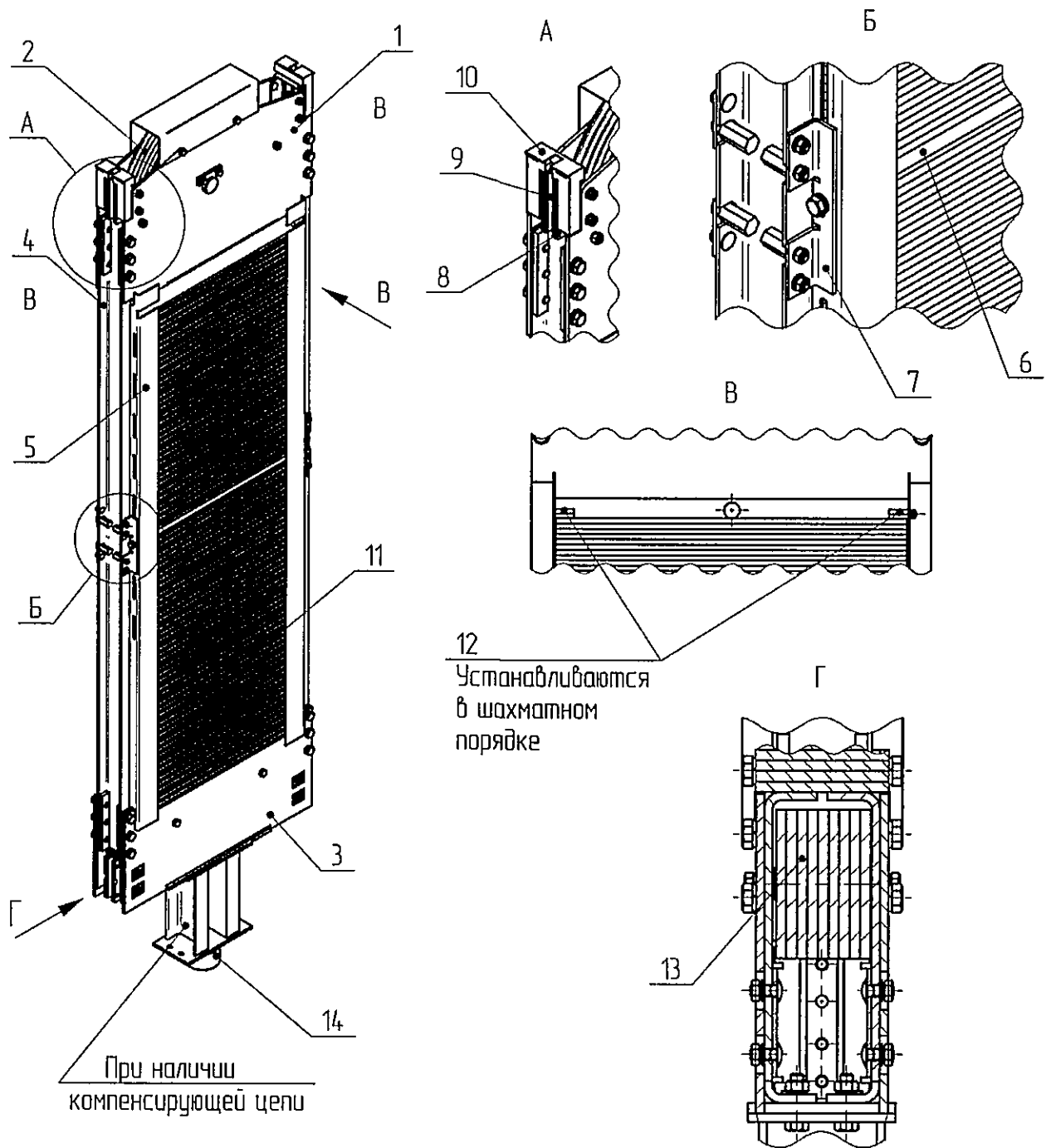
Рис 17 Противовес
