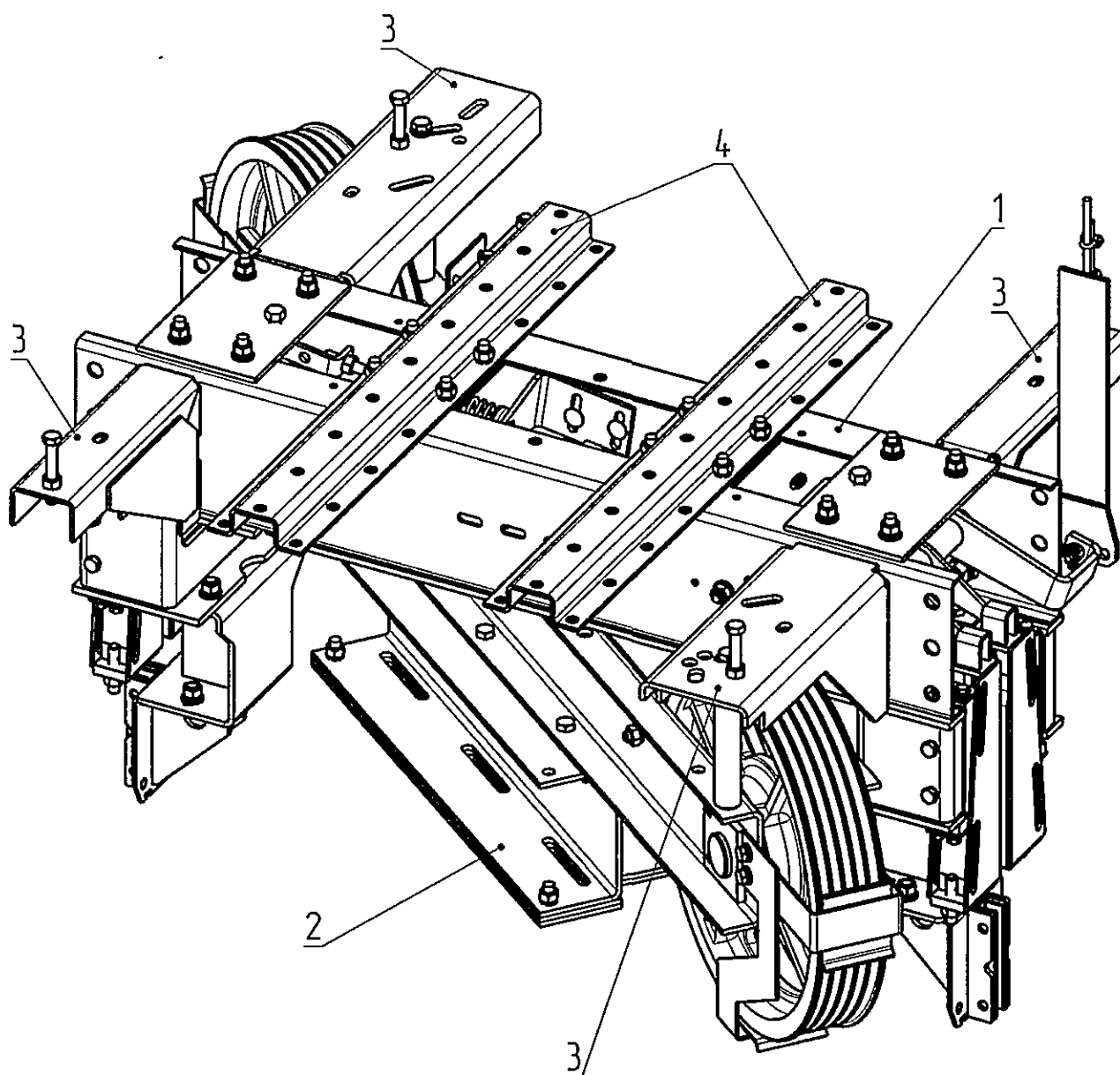
Рис. 11 Балка нижняя
