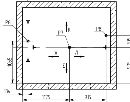
Схема расположения монтажных крюков над лифтовой шахтой
