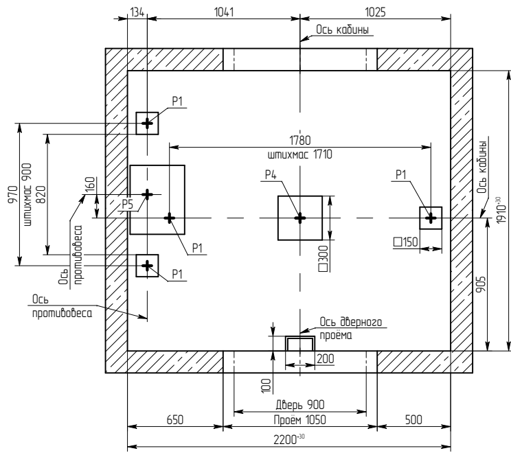
Б - Б (1:25) (1)
