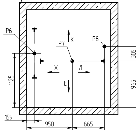
Схема расположения монтажных крюков над лифтовой шахтой
