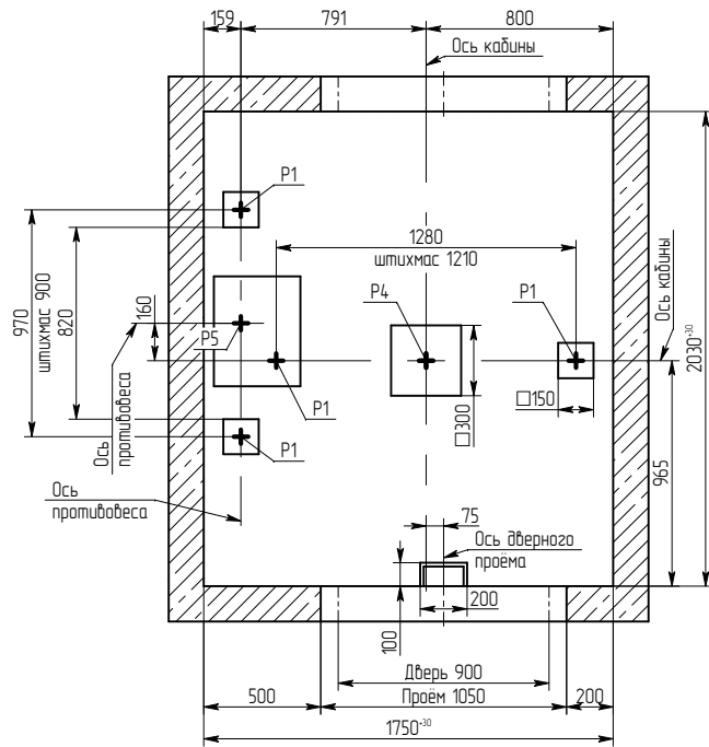
Б - Б (1:25) (1)
